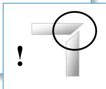
Bild 3: Isolierglas-Außenecke ohne Rahmen mit 45° Gehrung – die Ausführung der Außenecke als 45° Gehrung erfordert eine spezielle Kantenbearbeitung
